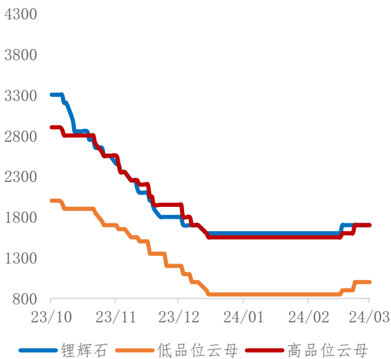
图 3：锂精矿价格（元/吨）
