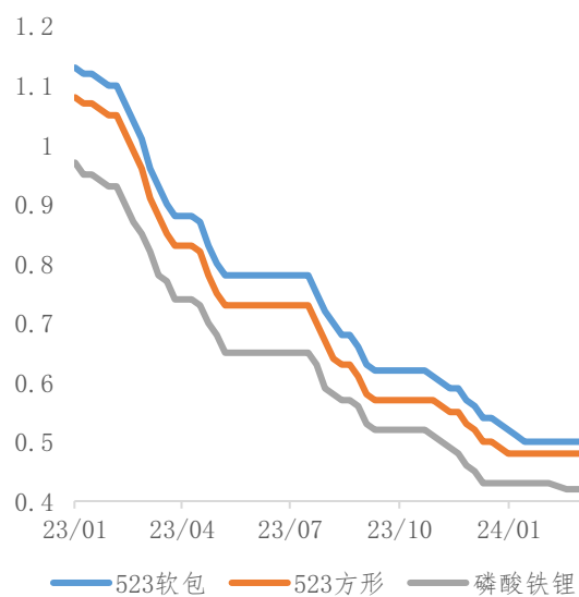
图 10：电芯售价 (元/Wh)
