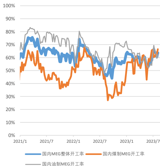
图 4：国内乙二醇装置开工率
